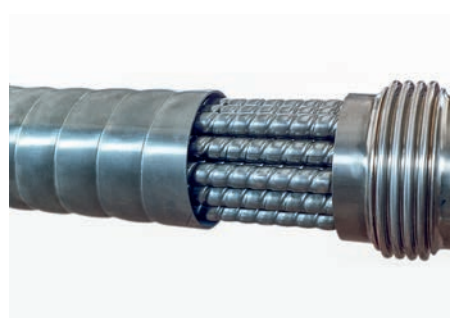
Wärmetauscher Industrie Cross Flo
